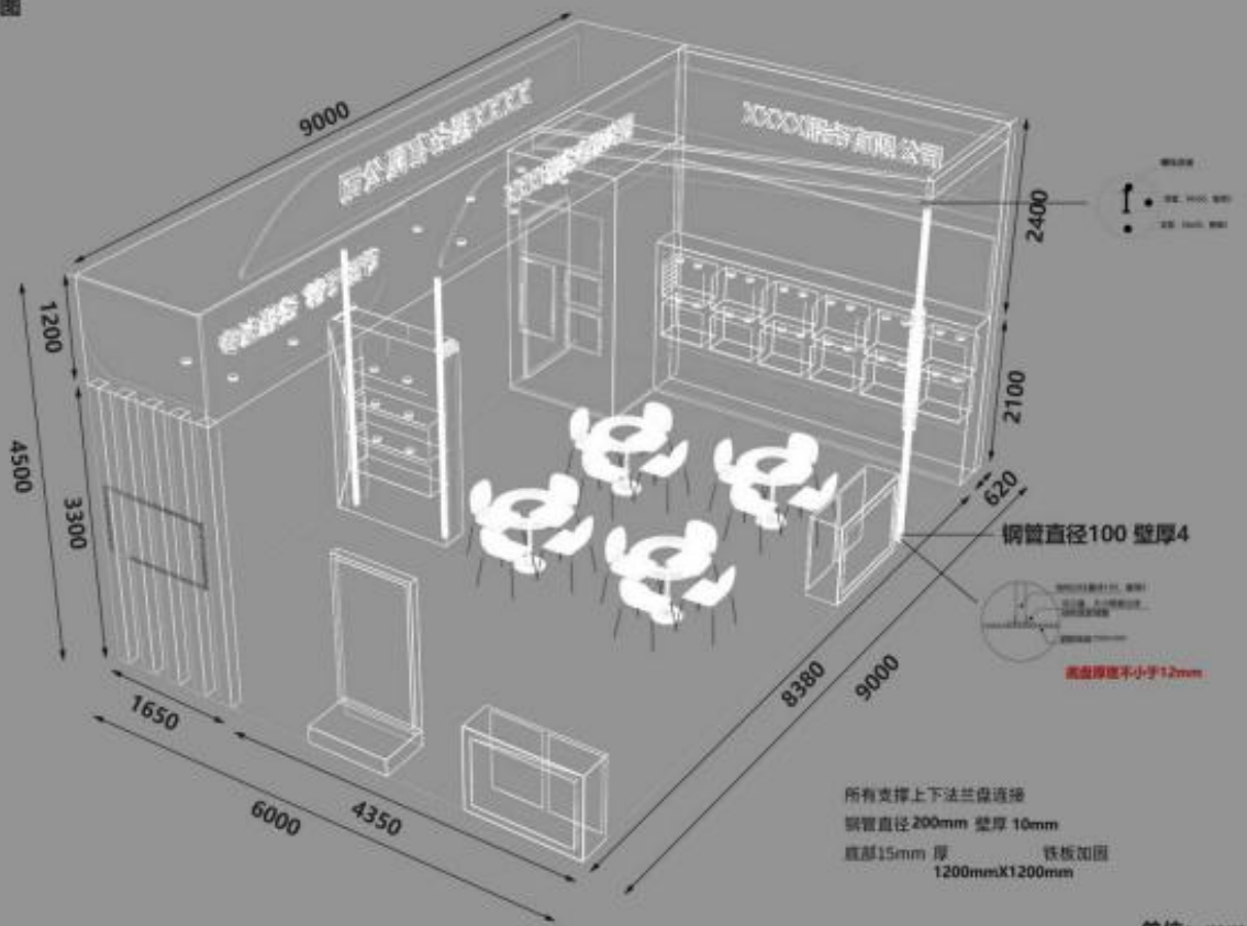
结构图
